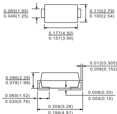
DO-214AC(SMA)
