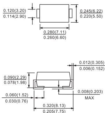
DO-214AB(SMC)
