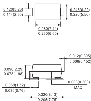
DO-214AB(SMC)
